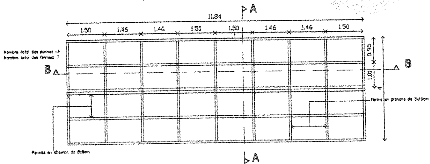
PLAN DE CHARPENTE
