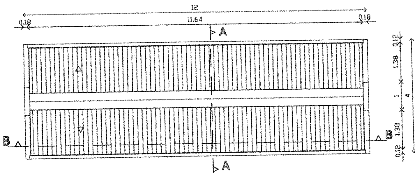
PLAN DE TOITURE
