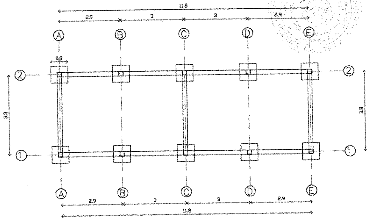
PLAN DE FONDATION
